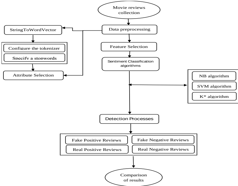
شكل (1) الخطوات والتقنيات المستخدمة في تحليل المشاعر
