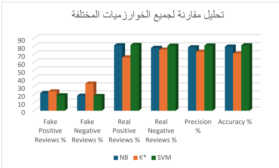
شكل (4) رسم بياني وضع تحليل مقارنة لثلاث خوارزميات
