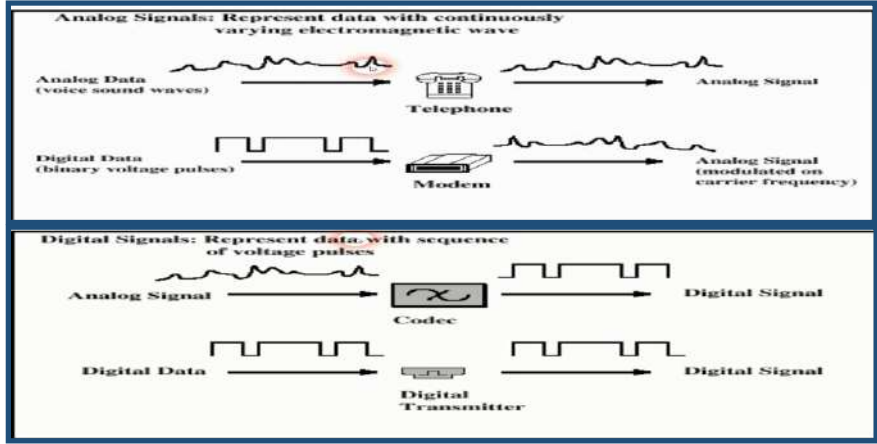
الشكل رقم (6) يوضح عمليات التحويل الاربعة للإشارات التناظرية والرقمية
